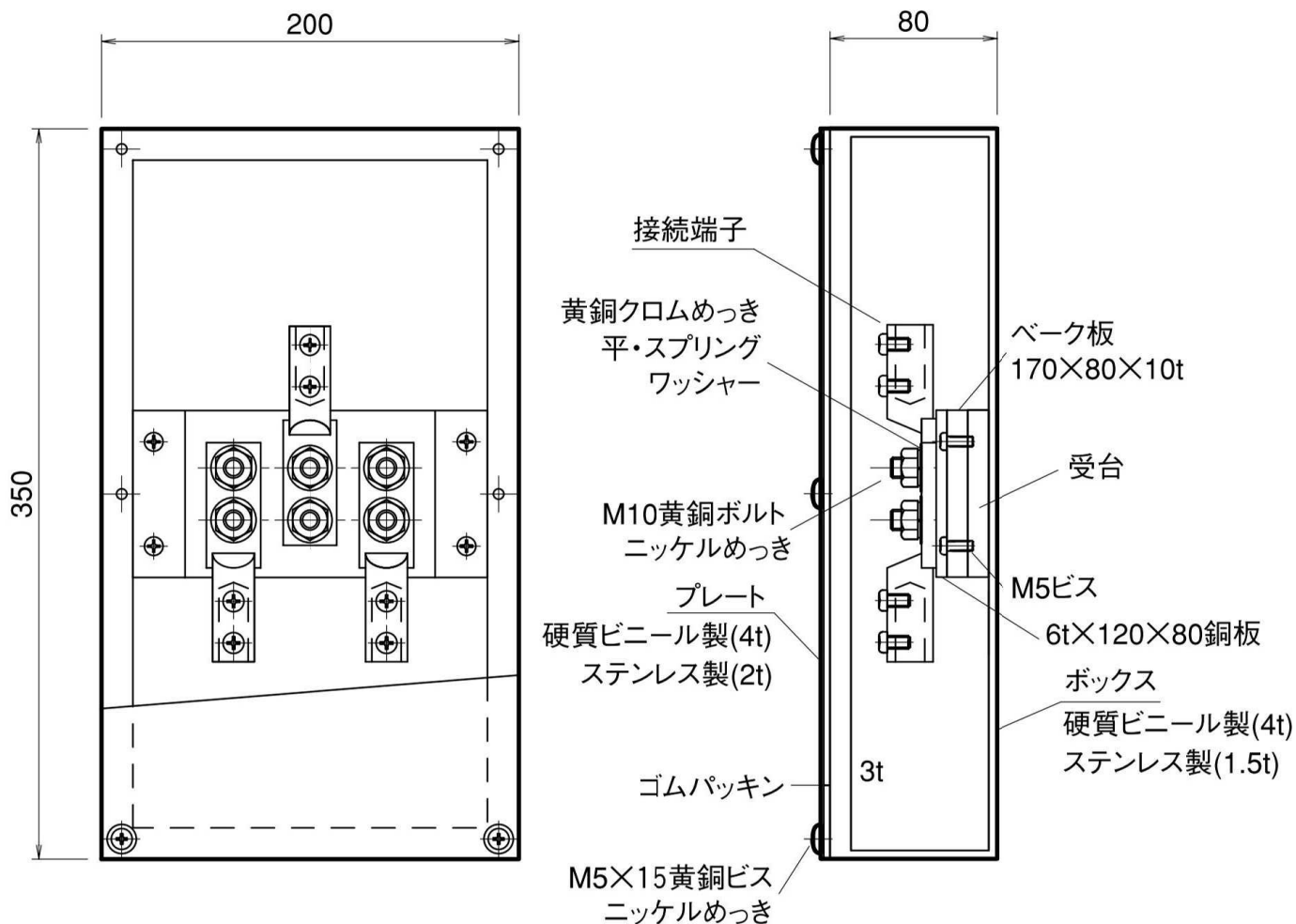
図はボックス硬ビ・プレート硬ビ製を示す 図は、細口端子使用例
